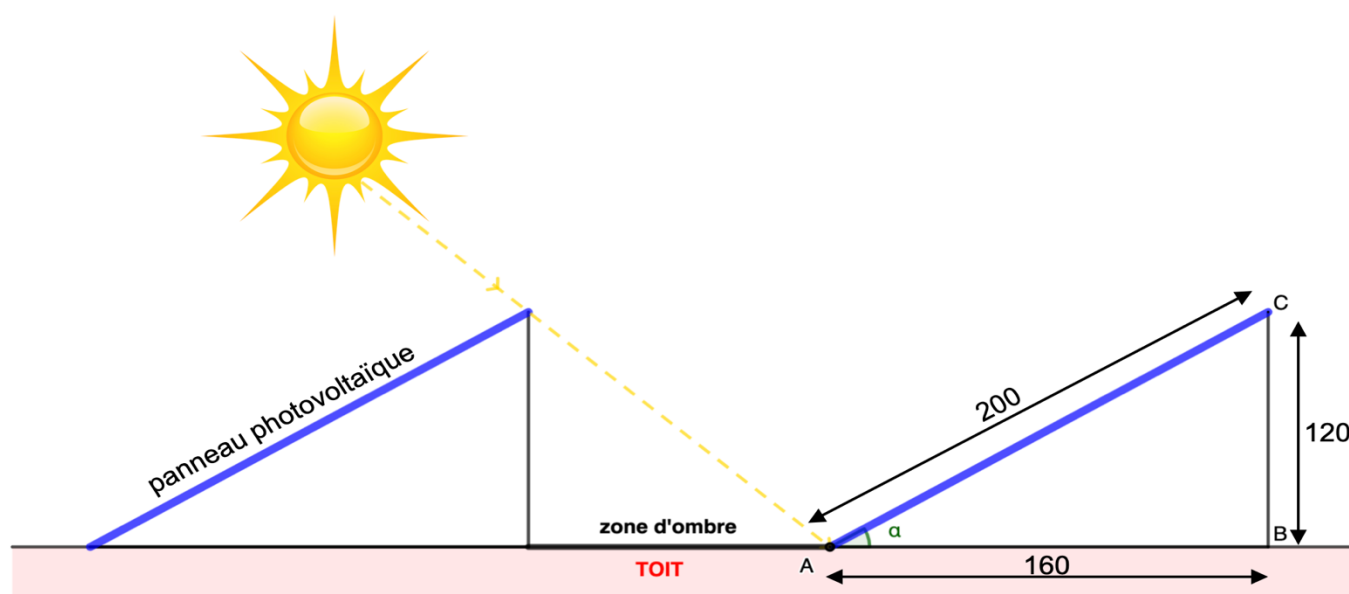
DOCUMENT 3 - Schéma de l'installation des supports des panneaux solaires (le dessin n'est pas à l'échelle, les mesures sont en cm)
